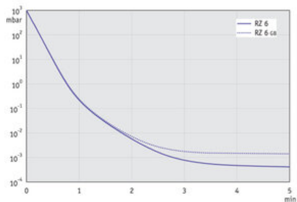
RZ 6 +FO +VS 16 +Set DCP+VSP 3000 - График: "Вакуумирование 10 л емкости" при 60 Гц
