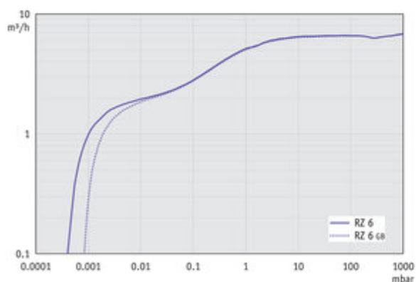
RZ 6 +FO +VS 16 +Set DCP+VSP 3000 - График: "Скорость откачивания при 60 Гц"
