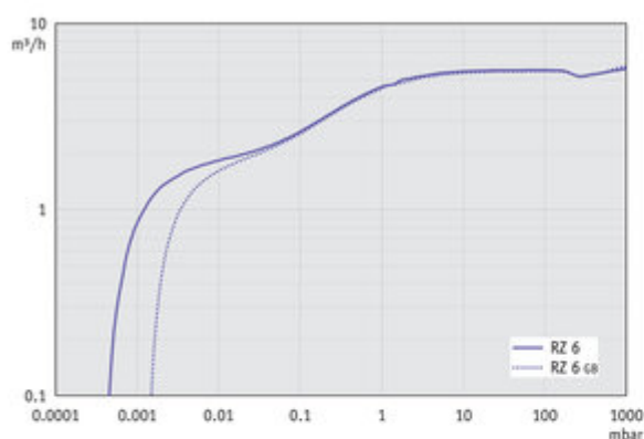
RZ 6 +FO +VS 16 +VACUU-VIEW extended - График: "Скорость откачивания при 60 Гц"
