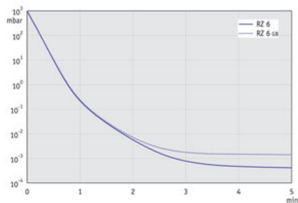
RZ 6 +FO +VS 16 +VACUU-VIEW extended - График: "Вакуумирование 10 л емкости" при 60 Гц
