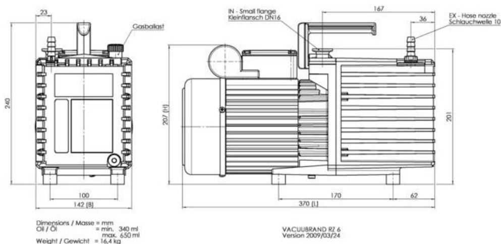
RZ 6 +FO +VS 16 - Габариты
