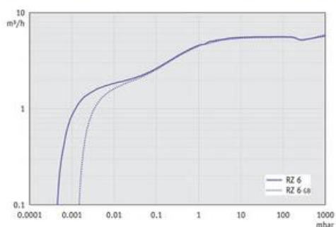
RZ 6 +FO +VS 16 - График: "Скорость откачивания при 60 Гц"
