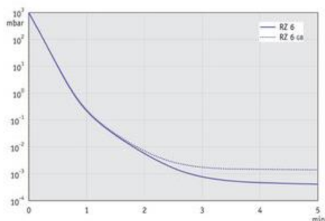
RZ 6 +FO +VS 16 - График: "Вакуумирование 10 л емкости" при 60 Гц
