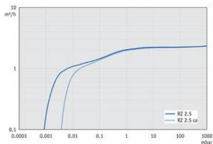
RZ 2.5 +FO +VS 16 - График: "Скорость откачивания при 50 Гц" RZ 2.5 +FO +VS 16 - График: "Вакуумирование 10 л емкости" при 50 Гц
