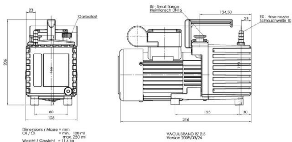
RZ 2.5 +FO +VS 16 - Габариты
