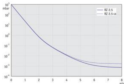
RZ 2.5 +FO +VS 16 - График: "Скорость откачивания при 60 Гц" RZ 2.5 +FO +VS 16 - График: "Вакуумирование 10 л емкости" при 60 Гц
