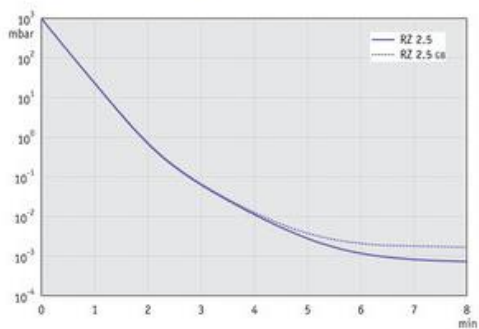
RZ 2.5 - График: "Вакуумирование 10 л емкости" при 60 Гц
