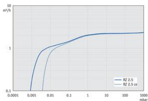
RZ 2.5 - График: "Скорость откачивания при 60 Гц"
