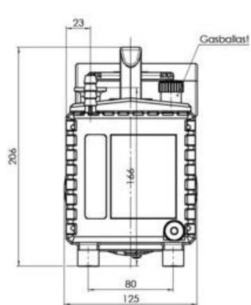
RZ 2.5 - Габариты
