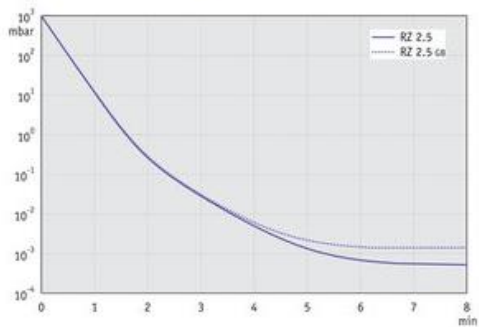
RZ 2.5 - График: "Вакуумирование 10 л емкости" при 60 Гц
