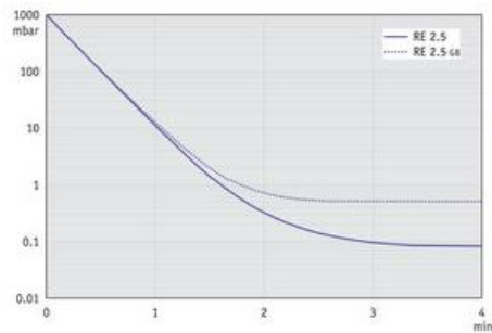
RE 2.5 - График: "Вакуумирование 10 л емкости" при 60 Гц
