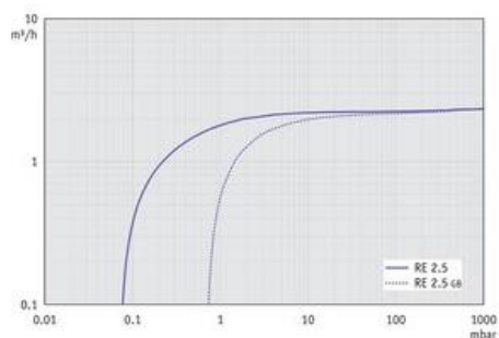
RE 2.5 - График: "Скорость откачивания при 60 Гц"
