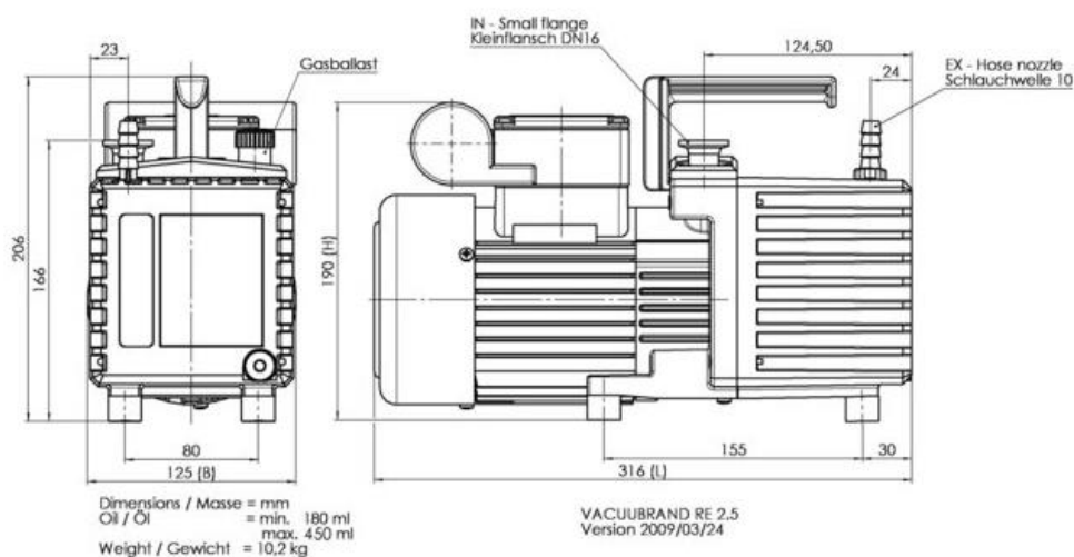
RE 2.5 - Габариты
