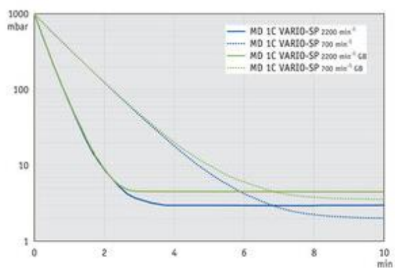
MD 1C VARIO-SP - График: "Вакуумирование 10 л емкости" при
