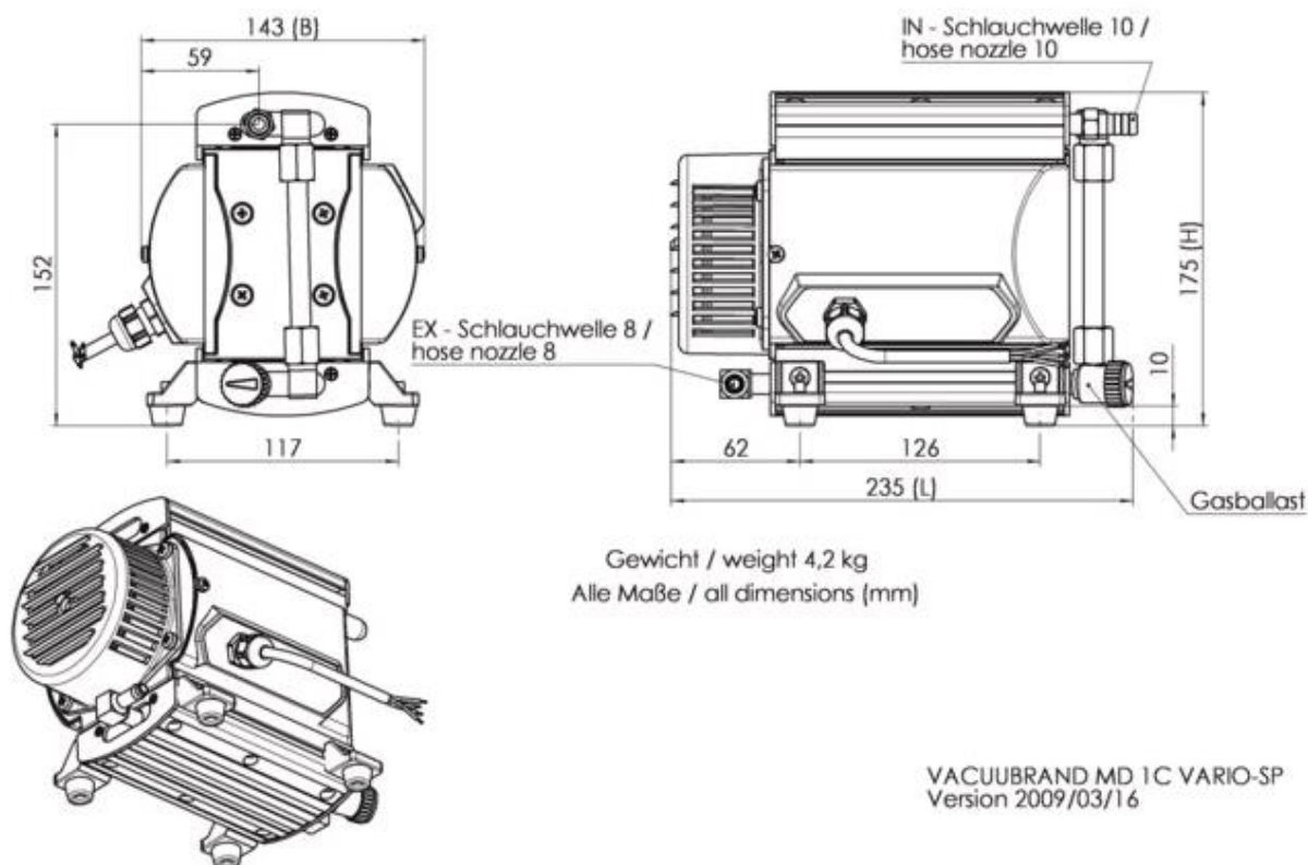
MD 1C VARIO-SP - Габариты
