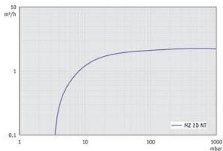
MZ 2D NT - График: "Скорость откачивания при 60 Гц"
