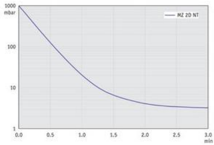
MZ 2D NT - График: "Вакуумирование 10 л емкости" при 60 Гц
