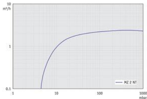
MZ 2 NT - График: "Скорость откачивания при 60 Гц"
