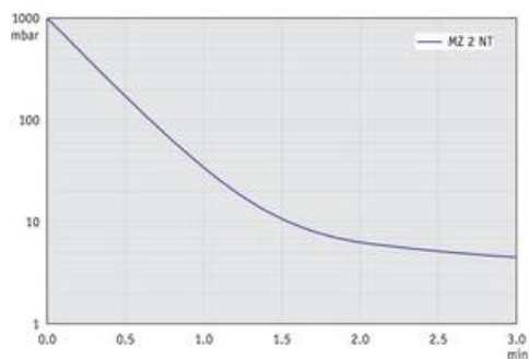
MZ 2 NT - График: "Вакуумирование 10 л емкости" при 60 Гц
