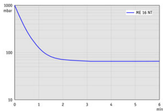
ME 16 NT - График: "Вакуумирование 100 л емкости" при 60 Гц
