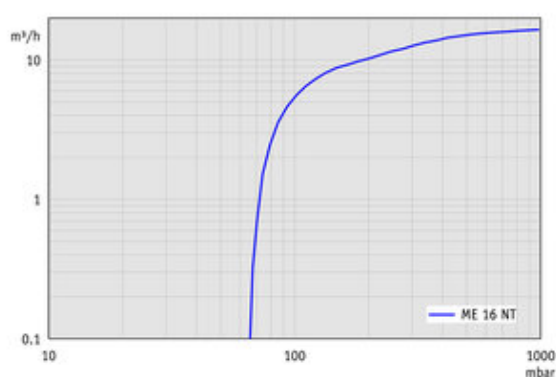
ME 16 NT - График: "Скорость откачивания при 60 Гц"
