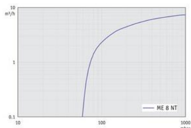
ME 8 NT - График: "Скорость откачивания при 60 Гц"
