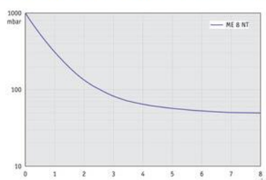
ME 8 NT - График: "Вакуумирование 100 л емкости" при 60 Гц
