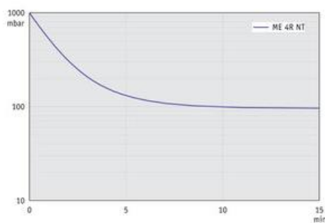
ME 4R NT - График: "Вакуумирование 10 л емкости" при 60 Гц
