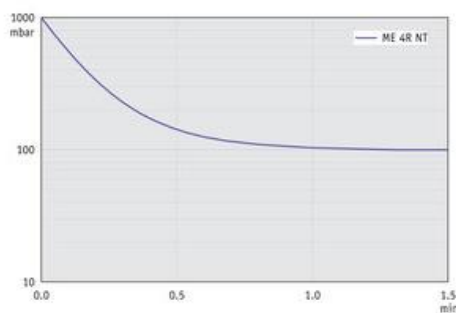
ME 4R NT - График: "Вакуумирование 10 л емкости" при 60 Гц
