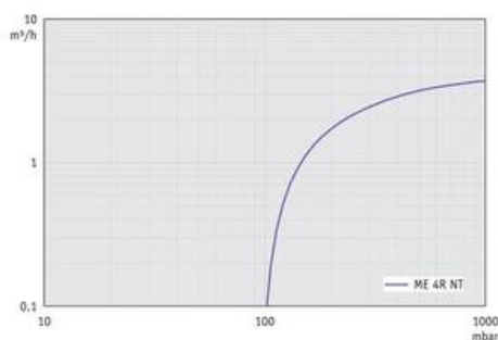
ME 4R NT - График: "Скорость откачивания при 60 Гц"
