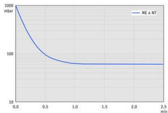
ME 4 NT - График: "Вакуумирование 10 л емкости" при 60 Гц
