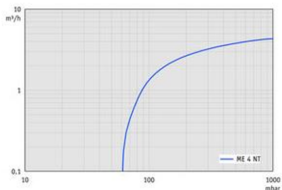
ME 4 NT - График: "Скорость откачивания при 60 Гц"
