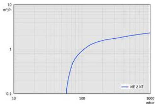
ME 2 NT - График: "Скорость откачивания при 60 Гц"
