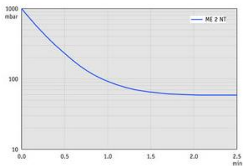
ME 2 NT - График: "Вакуумирование 10 л емкости" при 60 Гц
