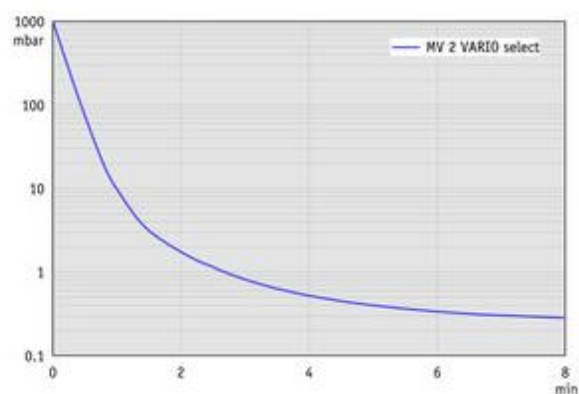
MV 2 VARIO select - График: "Вакуумирование 10 л емкости" при
