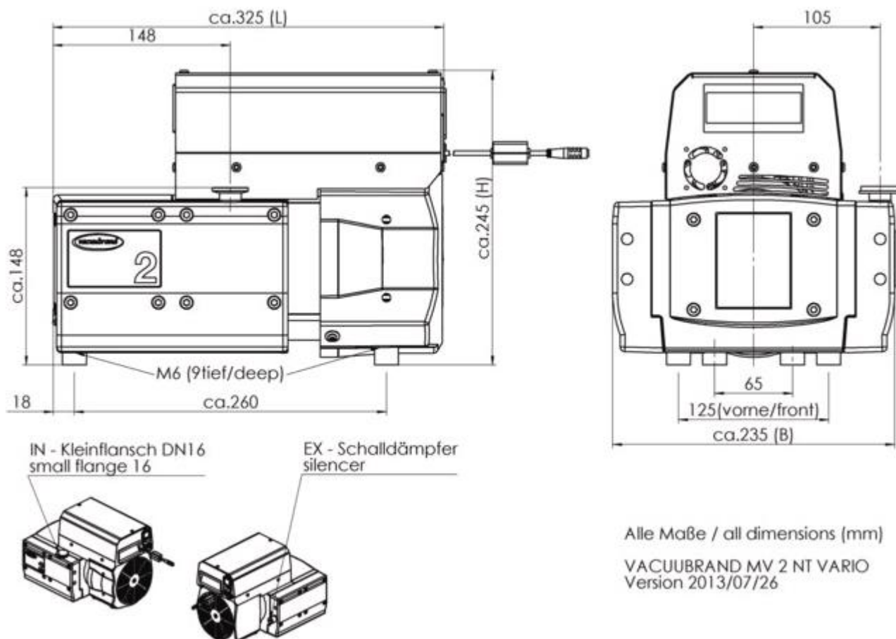
MV 2 VARIO select - Габариты
