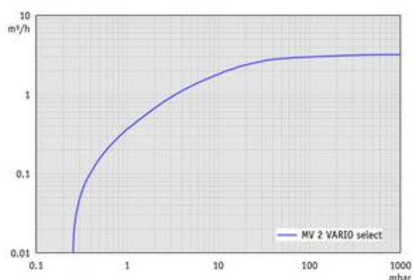
MV 2 VARIO select - График: "Скорость вакуумирования"
