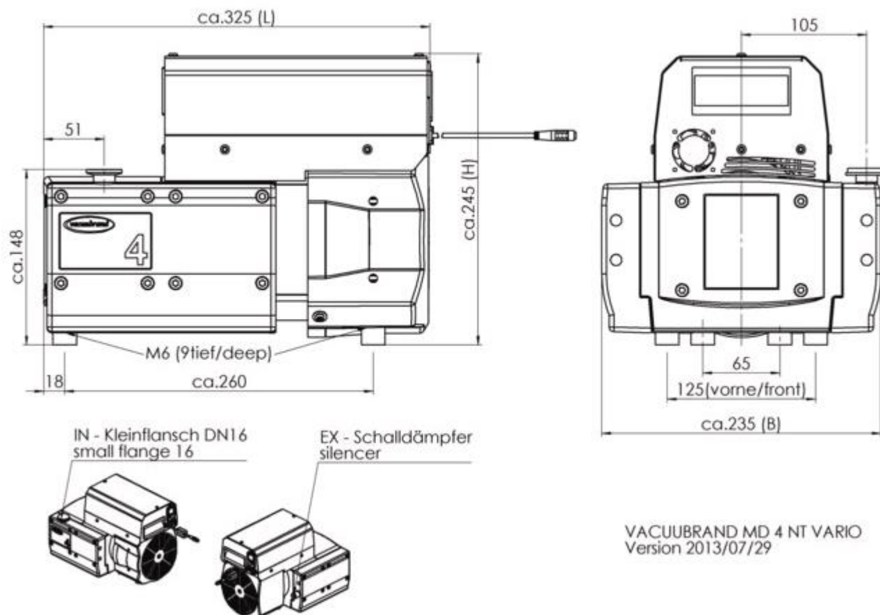
MD 4 VARIO select - Габариты
