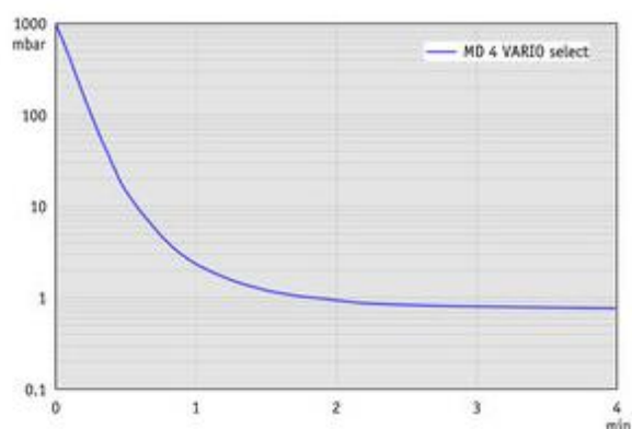
MD 4 VARIO select - График: "Вакуумирование 10 л емкости" при
