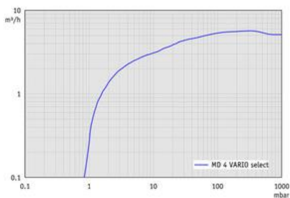
MD 4 VARIO select - График: "Скорость вакуумирования"
