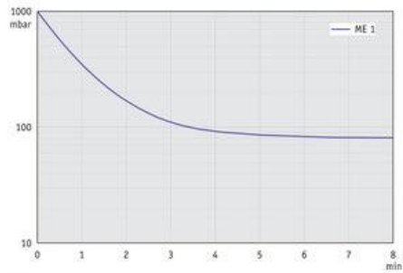
ME 1 - График: "Вакуумирование 10 л емкости" при 60 Гц
