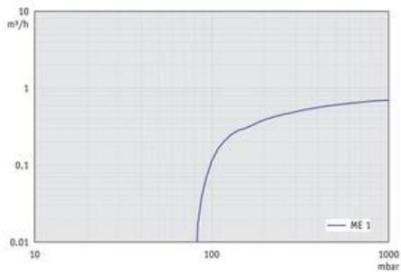
ME 1 - График: "Скорость откачивания при 60 Гц"
