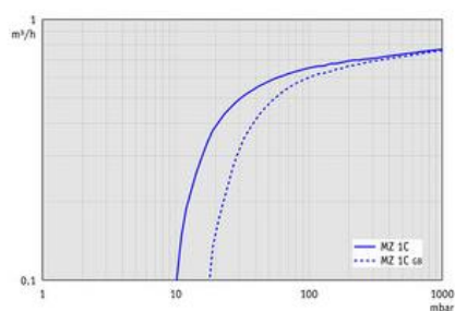
MZ 1C - График: "Скорость откачивания при 60 Гц"
