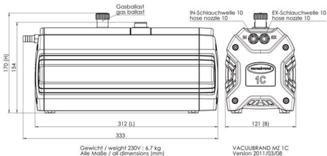
MZ 1C - Габариты
