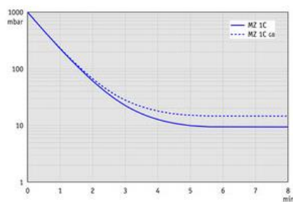
MZ 1C - График: "Вакуумирование 10 л емкости" при 60 Гц
