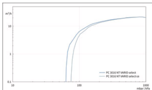
PC 3016 NT VARIO select - График: "Скорость вакуумирования" PC 3016 NT VARIO select - График: "Вакуумирование 100 л емкости"
