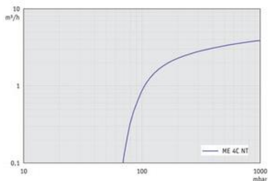
ME 4C NT - График: "Скорость откачивания при 60 Гц"
