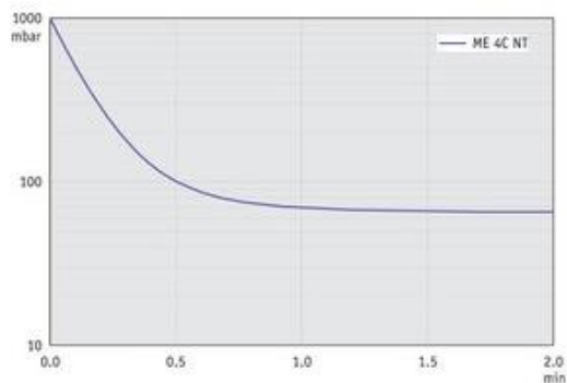
ME 4C NT - График: "Вакуумирование 10 л емкости" при 60 Гц
