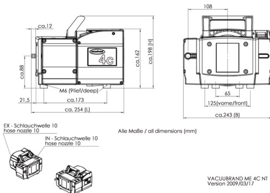
ME 4C NT - Габариты
