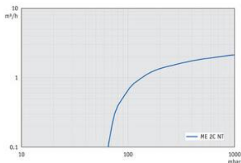
ME 2C NT - График: "Скорость откачивания при 60 Гц"
