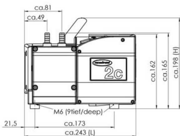
ME 2C NT - Габариты
