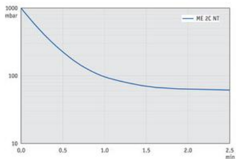
ME 2C NT - График: "Вакуумирование 10 л емкости" при 60 Гц
