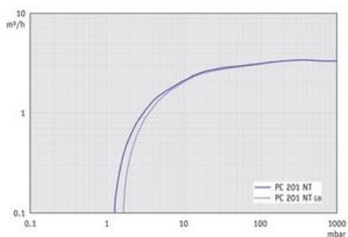
PC 201 NT - График: "Скорость откачивания при 60 Гц"
