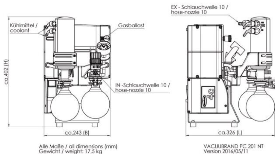
PC 201 NT - Габариты
