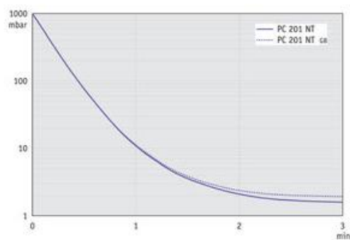
PC 201 NT - График: "Вакуумирование 10 л емкости" при 60 Гц
