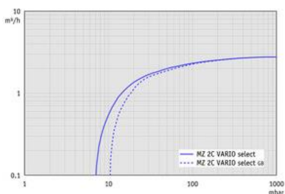
MZ 2C VARIO select - График: "Скорость вакуумирования"
