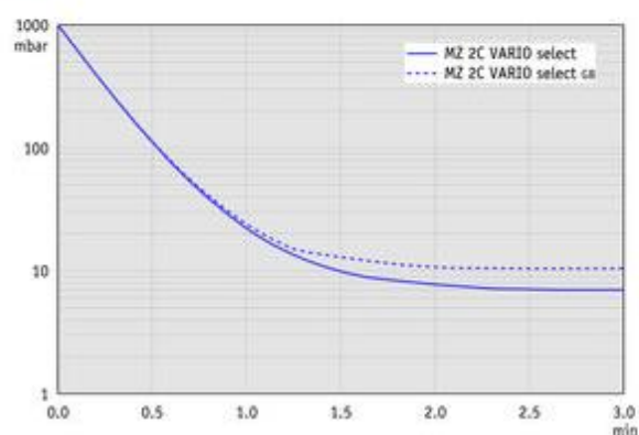
MZ 2C VARIO select - График: "Вакуумирование 10 л емкости" при
