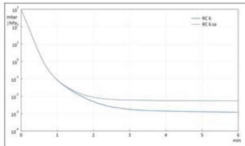
RC 6 - График: "Вакуумирование 10 л емкости" при 60 Гц
