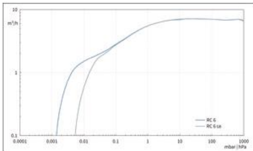
RC 6 - График: "Скорость откачивания при 60 Гц"
